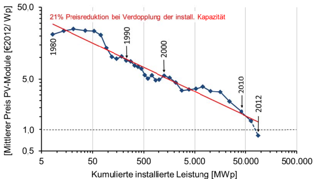
Abbildung 4: Historische Entwicklung der Preise für PV-Module (PSE AG/Fraunhofer ISE, Datenquelle: Strategies Unlimited/Navigant Consulting, 2012 geschätzt). Die Gerade zeigt den Trend der Preisentwicklung.
