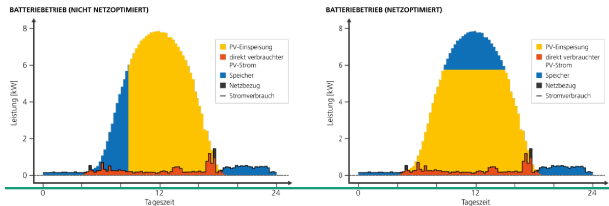
Abbildung 54: Gegenüberstellung der konventionellen und der netzdienlichen Betriebsführung [ISE7]
