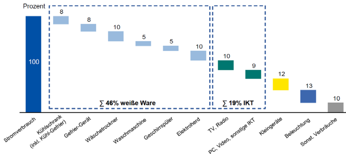
Abbildung 52: Stromverbrauch eines durchschnittlichen Haushalts ohne Warmwasseraufbereitung, aus [RWE]
