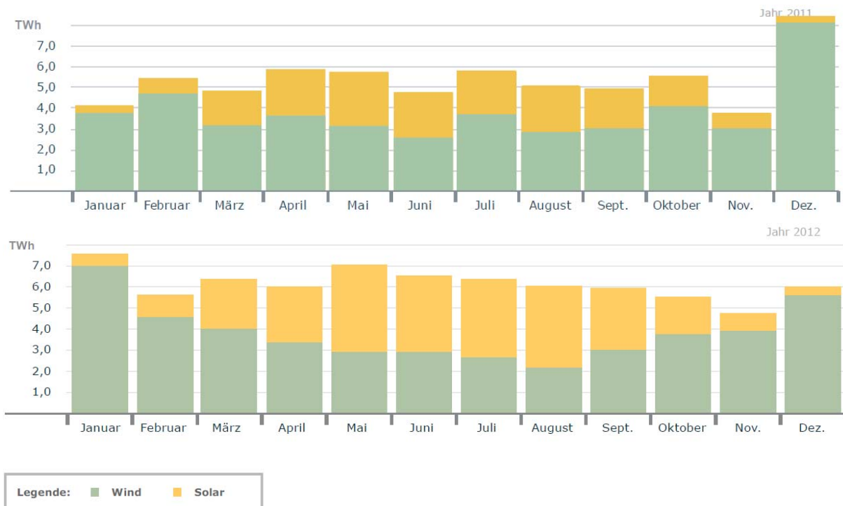
Abbildung 29: Monatliche PV- und Windstromproduktion der Jahre 2011-2012 [ISE4]
