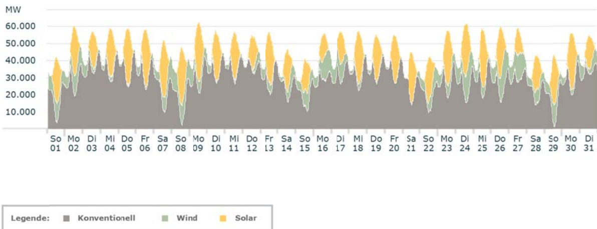
Abbildung 48: Simuliertes Last- und Stromerzeugungsprofil auf Basis beispielhafter Wetterdaten für eine sonnige Maiwoche bei installierten Leistungen von 50 GW PV und 40 GW Wind, die Spitzenleistungen von 35 GW PV und 21 GW Wind liefern (B. Burger, Fraunhofer ISE)
