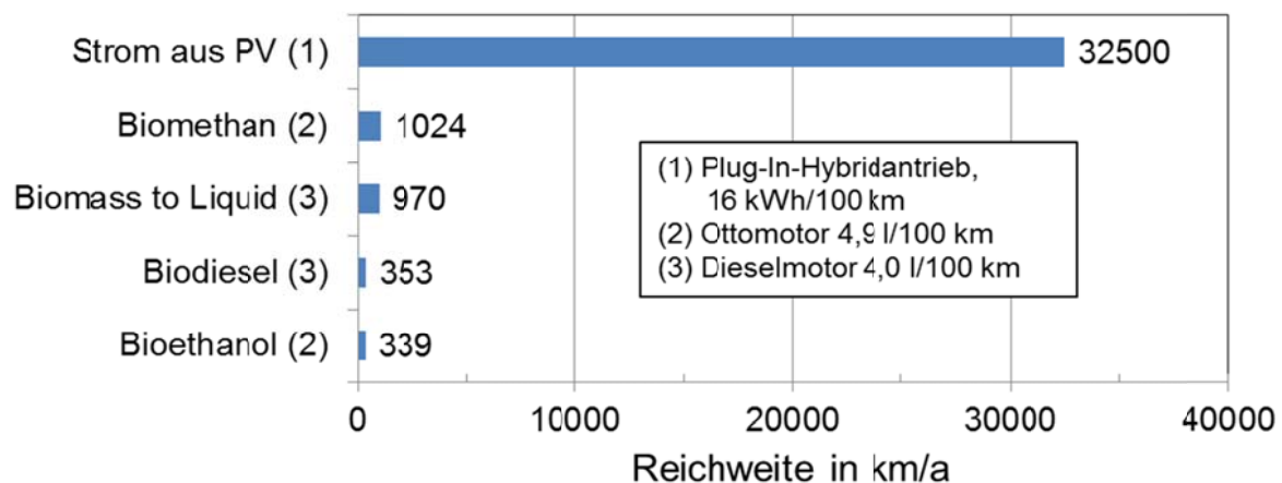
Abbildung 30: Fahrzeugreichweite mit dem Jahresertrag von 1 a = 100 m 2 Energiepflanzenanbau (2,3) und von 40 m 2 PV-Modulen, aufgeständert auf 100 m 2 ebener Grundfläche, Quellen: Photon, April 2007 (1) und Fachagentur Nachwachsende Rohstoffe (2), (3)
