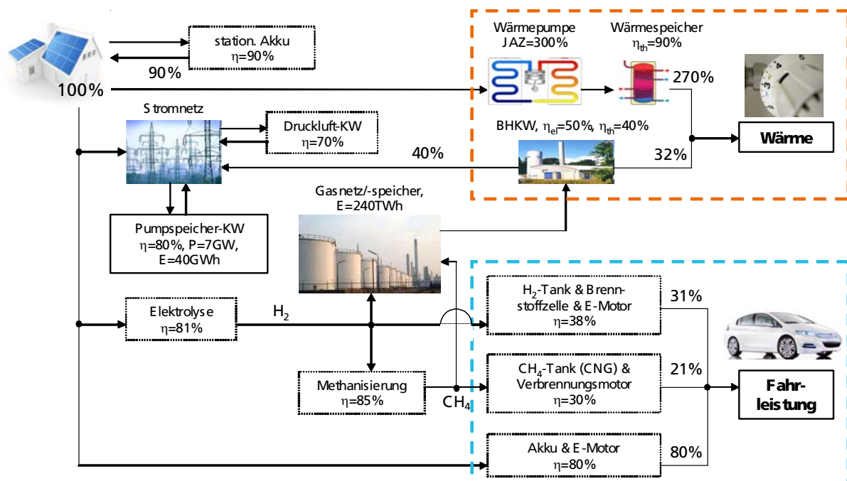
Abbildung 55: Mögliche Pfade zur Wandlung und Speicherung von PV-Strom mit orientierenden Angaben zu Wirkungsgraden
