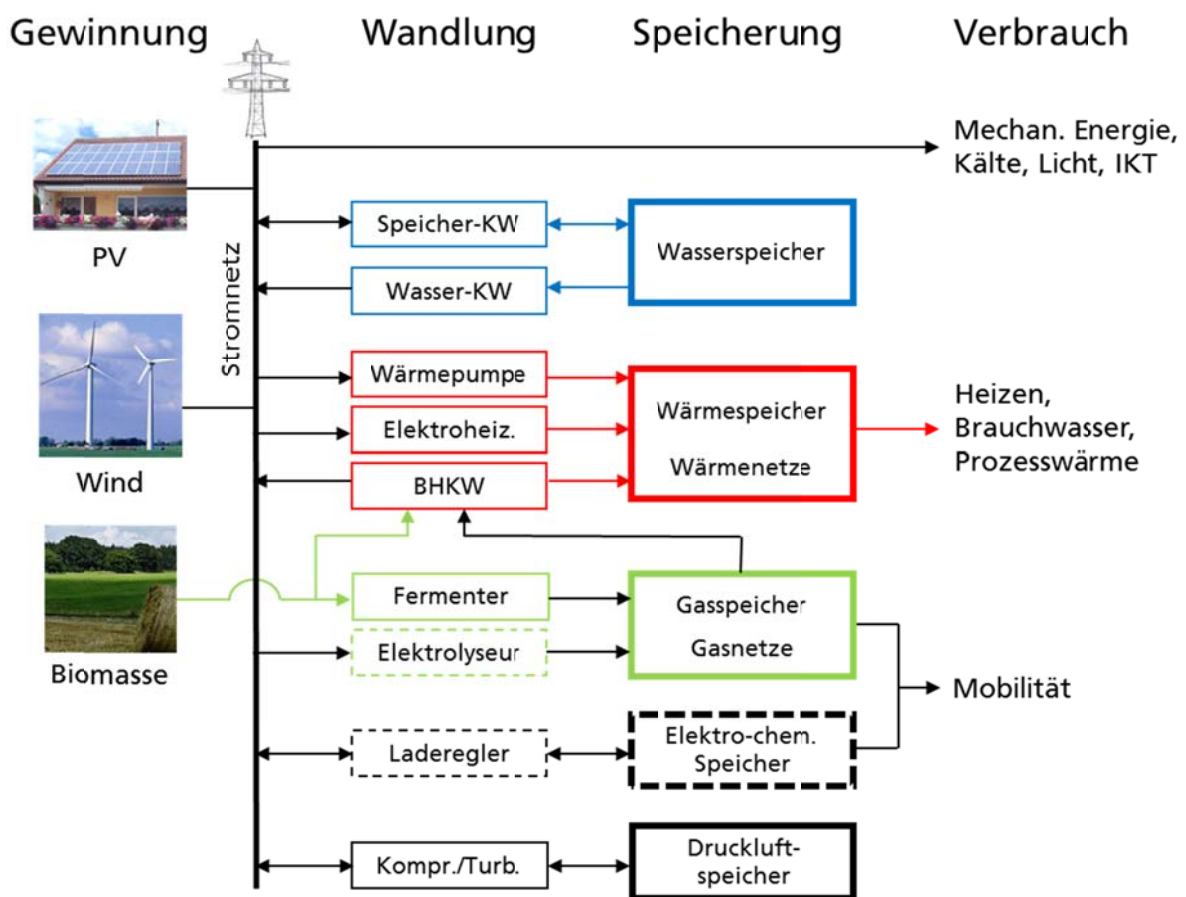
Abbildung 35: Vereinfachte schematische Darstellung eines Erneuerbaren Energiesystems mit den wichtigsten stromnetzgebundenen Bausteinen der Kategorien Gewinnung, Wandlung, Speicherung und Verbrauch; IKT: Informations- und Kommunikationstechnik; gestrichelte Kästen: zur Zeit noch sehr geringe Leistungen/Kapazitäten verfügbar
