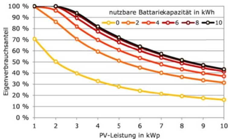
Abbildung 53: Eigenverbrauchsanteil in Abhängigkeit von Batteriekapazität und Leistung des Solargenerators für einen Einfamilienhaushalt mit einem Jahresstromverbrauch von 4.700 kWh. [Quasch]
