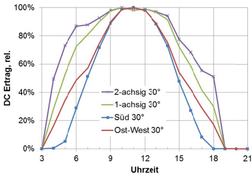
Abbildung 49: Stromertragsprofile von PV-Anlagen in verschiedenen Montagevarianten, berechnet mit der Software PVsol für einen überwiegend klaren Julitag am Standort Freiburg
