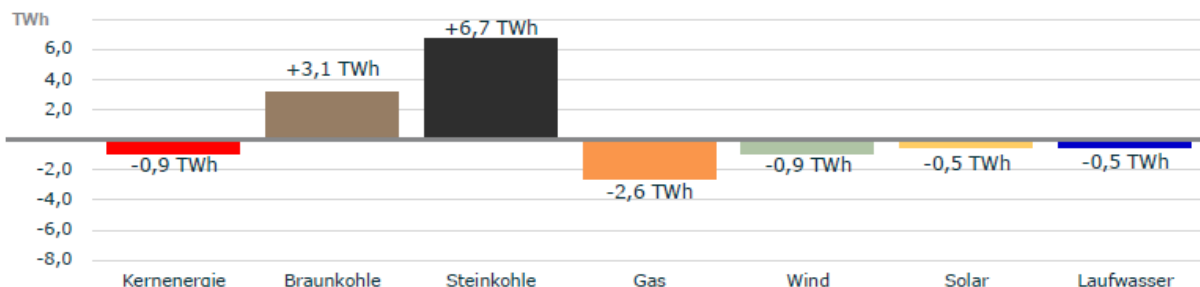
Abbildung 20: Veränderung der Stromerzeugung im ersten Quartal 2013 gegen 2012, die zusätzliche Produktion durch Braun- und Steinkohle wurde fast vollständig exportiert [ISE4]
