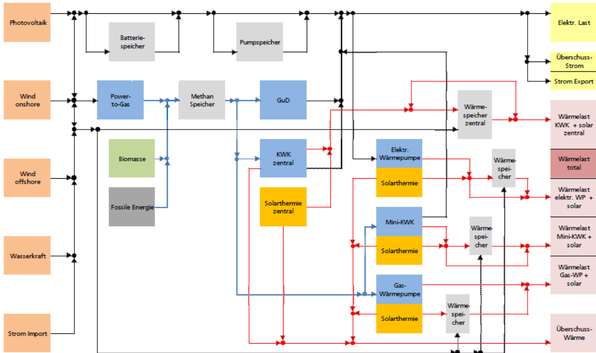
Abbildung 37: Szenario eines deutschen Energiesystems, schematische Darstellung der Systemzusammensetzung. [ISE5]
