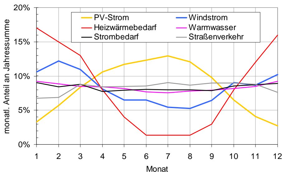
Abbildung 45: Grobe Abschätzung der monatlichen Verteilung (Jahressumme = 100%) für Sonnenstrom, berechnet für den Standort Freiburg aus [PVGIS], des Windstroms [DEWI], des Heizwärmebedarfs nach Gradtagszahlen (VDI 2067 bzw. DIN 4713), des Energiebedarfs für die Warmwasserbereitung der Haushalte, des Strombedarfs [AGEB1] und des Kraftstoffabsatzes [MWV]
