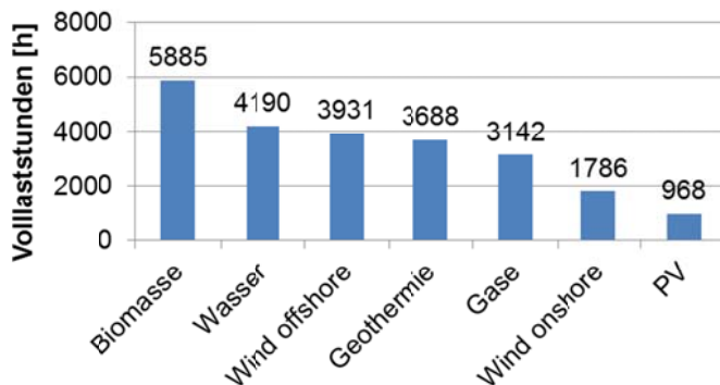
Abbildung 31: Prognostizierte Vollbenutzungsstunden für ganzjährig betriebene Anlagen, gemittelte Werte für die Jahre 2012 bis 2016, Daten aus [R2B]
