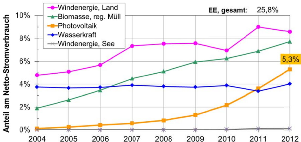
Abbildung 1: Entwicklung des Anteils Erneuerbarer Energien am Netto-Stromverbrauch (Endenergie) in Deutschland, Daten aus [BMW1], [BDEW3], [BDEW4], [BMU4]
