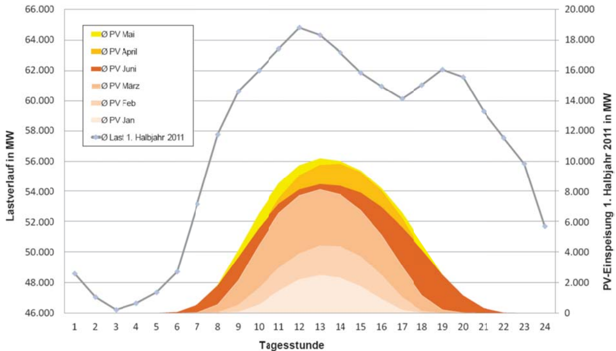
Abbildung 47: Durchschnittliches Lastprofil und durchschnittliche monatliche PV-Einspeisepprofile im ersten Halbjahr 2011 [IZES]
