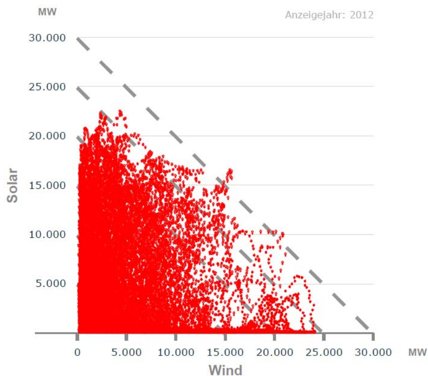
Abbildung 28: Mittlere Stundenleistung für die Einspeisung von Sonnen- und Windstrom im Jahr 2012 [ISE4]
