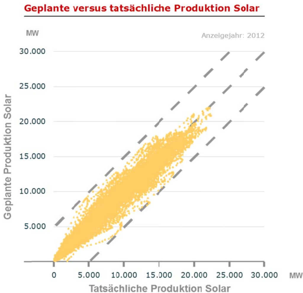
Abbildung 27: Stündliche tatsächliche und geplante Stromproduktion im Jahr 2012 [ISE4]
